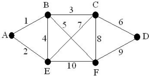
Fig. 1. Subnet
